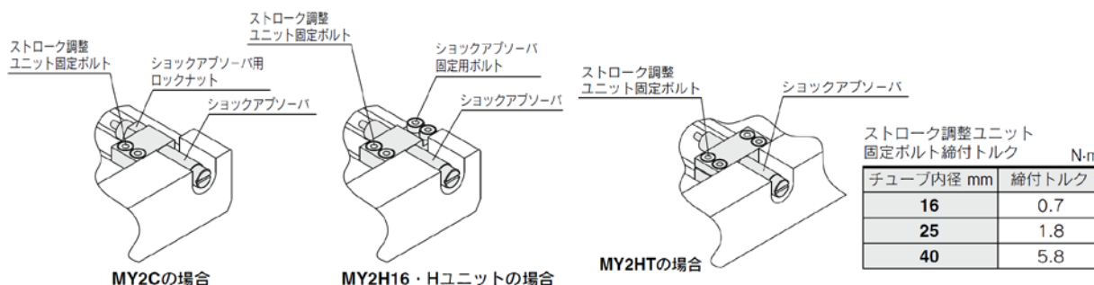
図-10. ストローク調整ユニット
