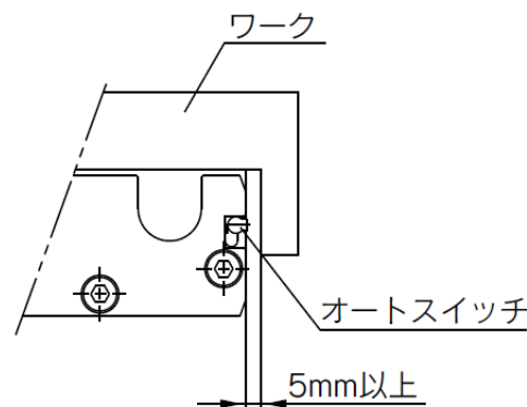
図-14 ガイド側取付の場合
