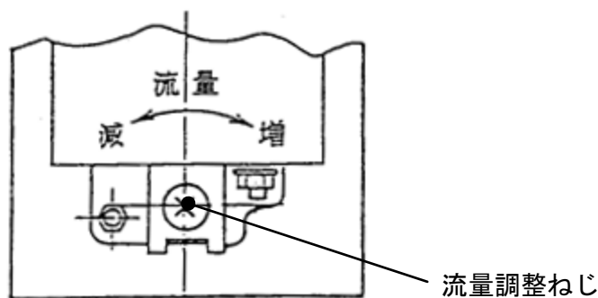
カバー取外し後の上面図
