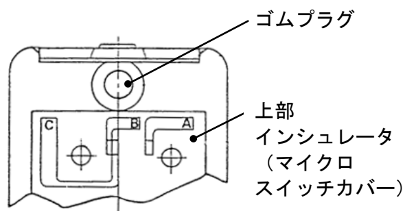
カバー取外し後の内部
