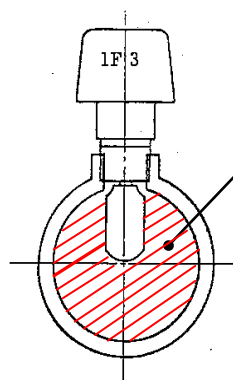
流量通過断面
