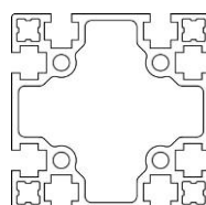
AFS-6060L-6
