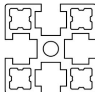
AFS-3060F-6
