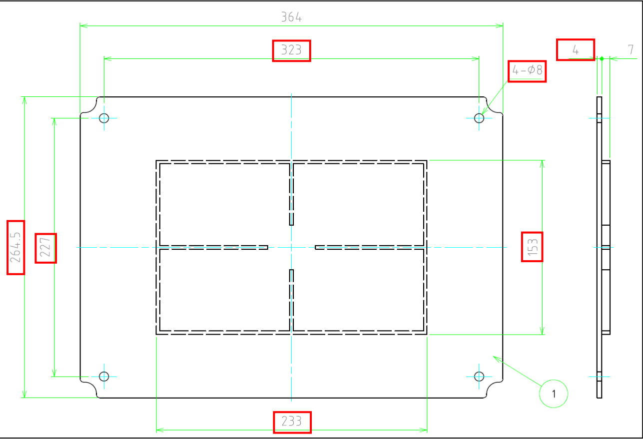
従来品の製品サイズ、寸法
