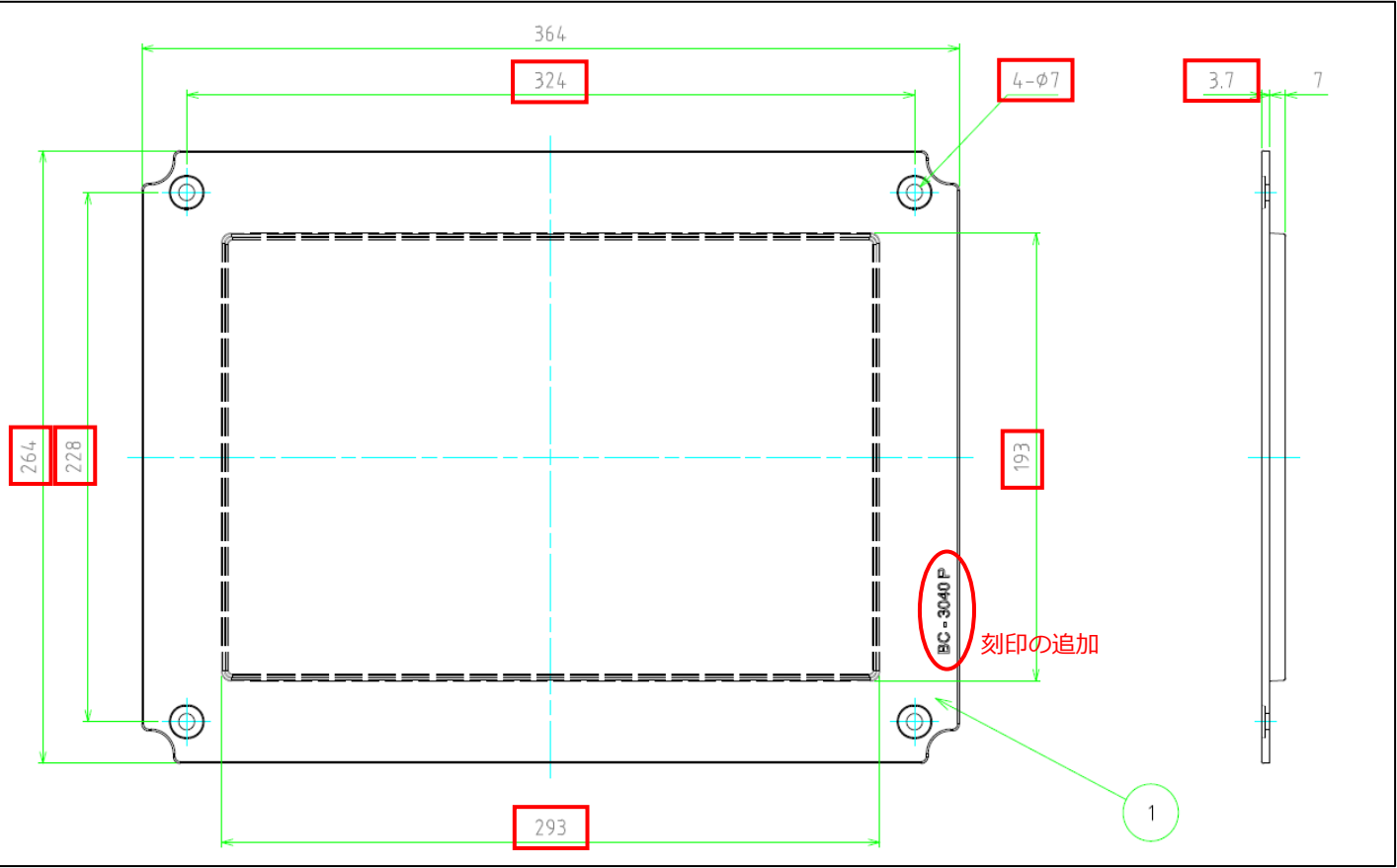
変更品の製品サイズ、寸法
