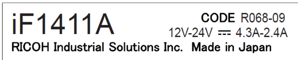
図 2-8 定格銘板イメージ(R068-09)
