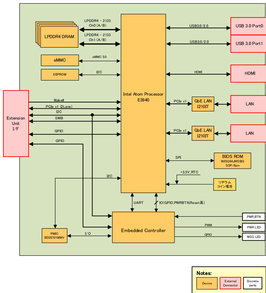
図 2-1 コントローラ全体ブロック図
