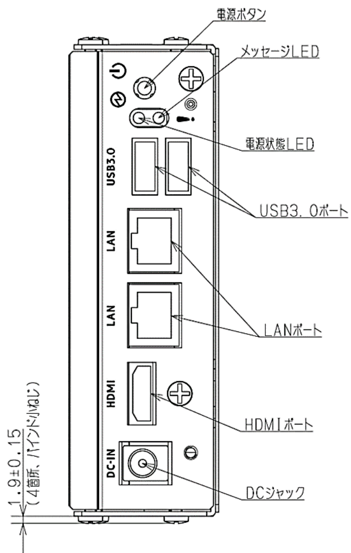
図 2-2 ポート配置図
