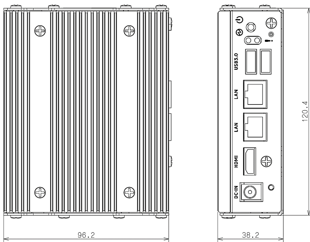
図 2-1 外形寸法図
