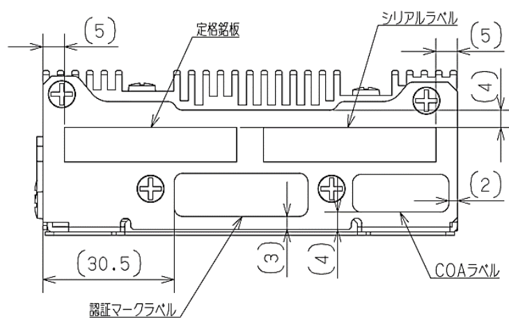
図 2-12 ラベル貼り付け位置
