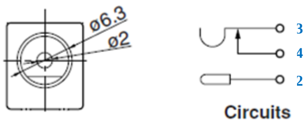
図 2-6 電源端子
