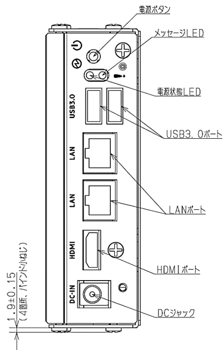
図 2-2 システム外観(正面)
