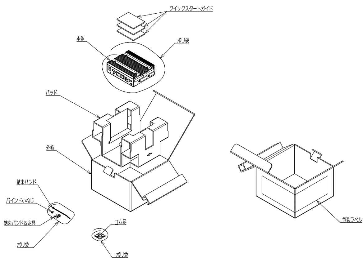
図 4-1 本体包装図
