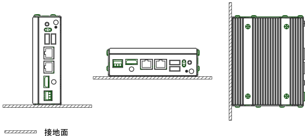
図 3-1 設置例
