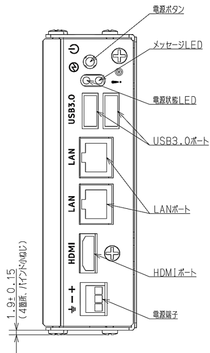
図 2-2 システム外観(正面)
