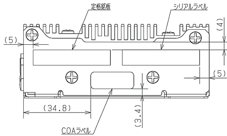
図 2-11 ラベル貼り付け位置
