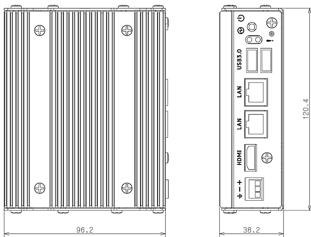
図 2-1 外形寸法図
