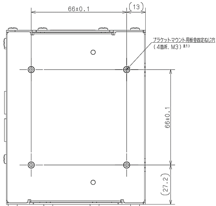
図 2-2 システム外観(正面)
