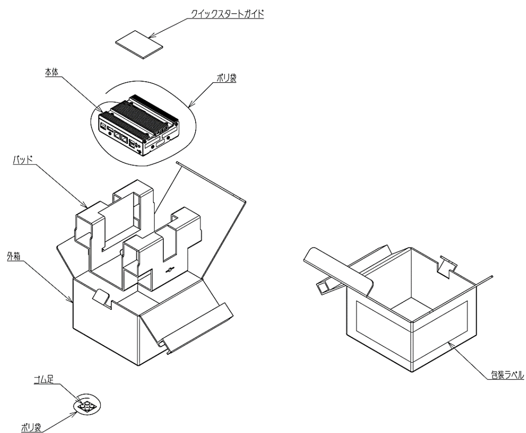
図 4-1 本体包装図
