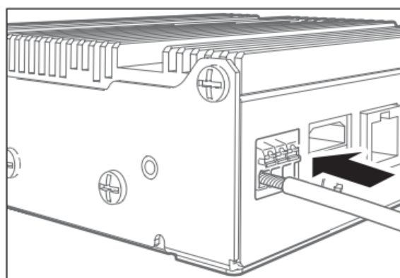
図 5-1 電線の接続
