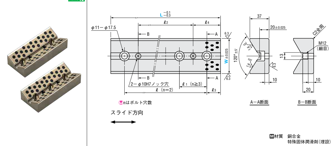
カムボトムガイドプレート RoHS10 CBGL
