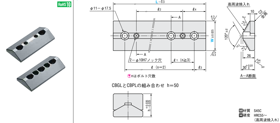
カムボトムスライドプレート RoHS10 CBPL
