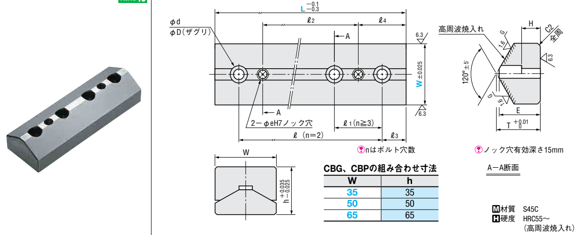
カムボトムスライドプレート RoHS10 CBP
