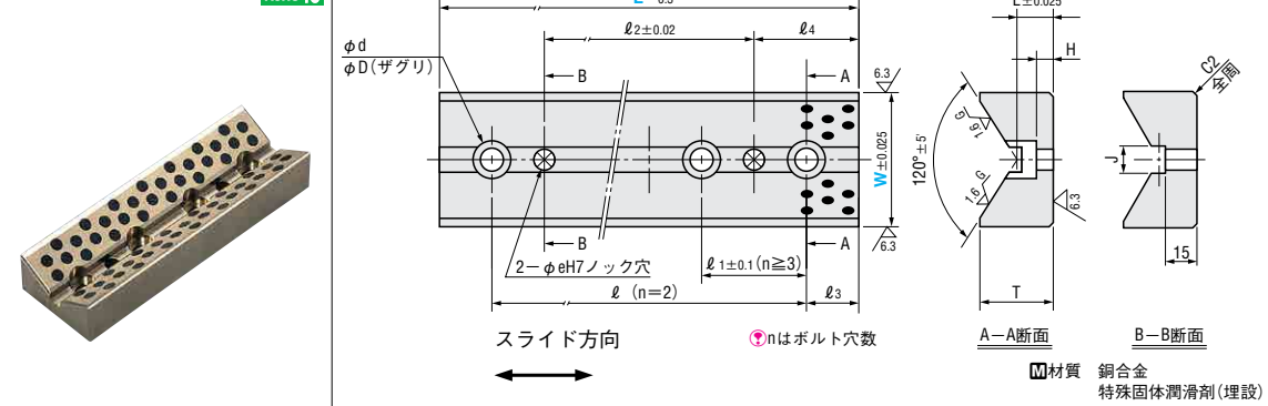
カムボトムガイドプレート RoHS10 CBG
