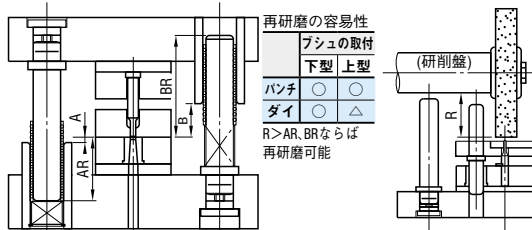
図1.下型ブシュと通常のブシュ
