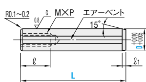
MSTP (タップ付精級タイプ)
