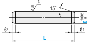
MSV (高精度タイプ)
