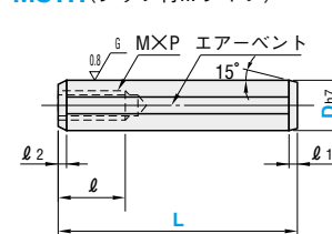
MSTH (タップ付h7タイプ)
