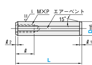
MSTM (タップ付m6タイプ)
