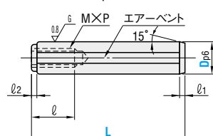
MSTM (タップ付m6タイプ)
