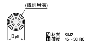
MTT (タップ付テーパタイプ)
