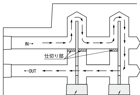
冷却用水穴(横穴)の先にエジェクタピンや傾斜スライドがあり、横穴が貫通できない場合、縦方向の水穴内を仕切り、バッフル板途中に穴を設けることで、IN-OUTを同一面上に設置する構造がとれます。
