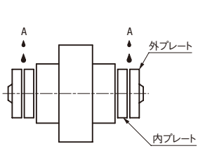
■図2:エンブラローラの場合
