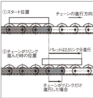
■搬送時のチェーンとパレットの関係
