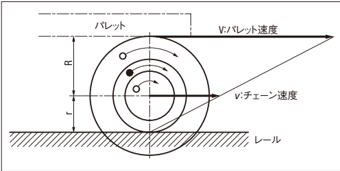
■搬送時のチェーンとパレットの関係
