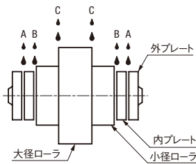
■図1:スチールローラの場合
