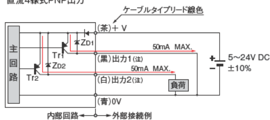
直流4線式PNP出力
