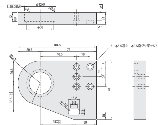
PLHDB-RE-FJ-R
