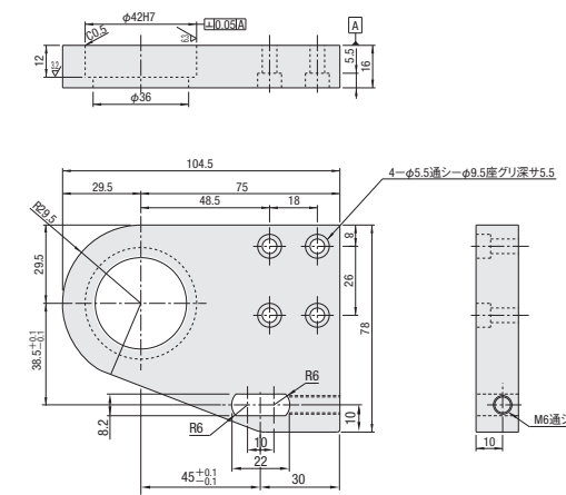
PLHDB-RE-FJ-R
