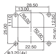
パネル穴あけ寸法
