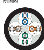
ケーブル断面図
