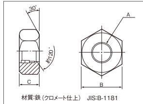
材質:鉄(クロメート仕上) JIS-B-1181
