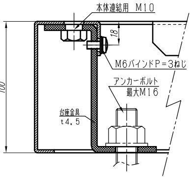
【台座金具取付詳細】
