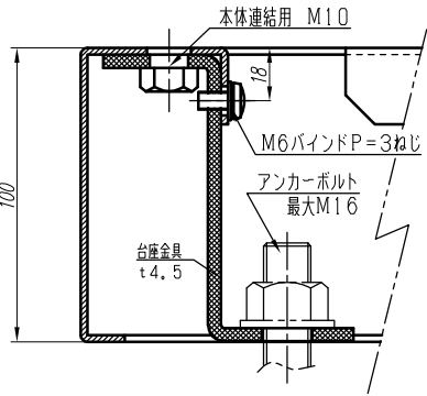
【台座金具取付詳細】
