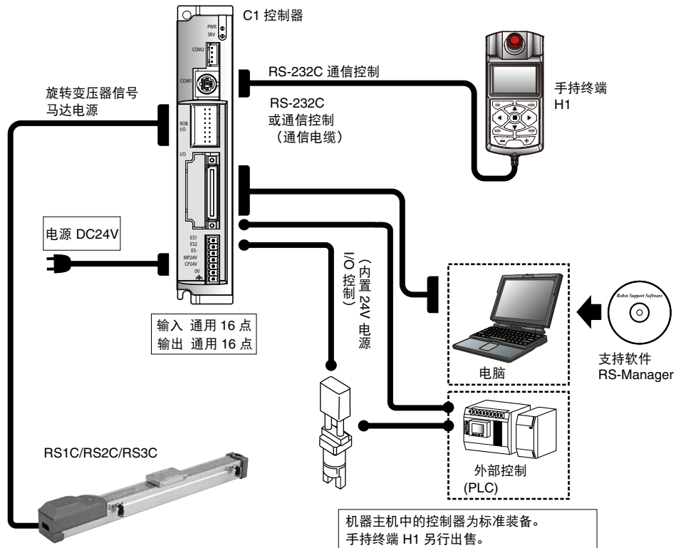
机器人的系统构成图 RS1C/RS2C/RS3C
