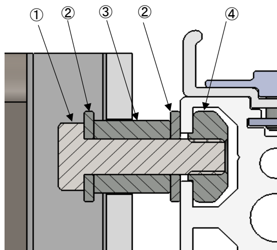
※印部説明図（断面図）
