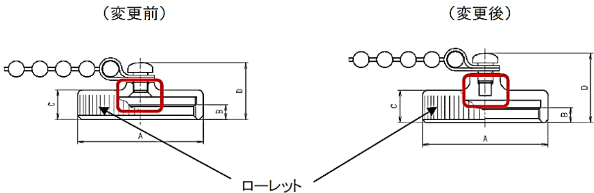
▼寸法比較表
