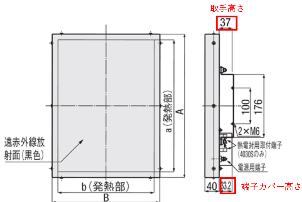
図 2 : 外形図 修正後
