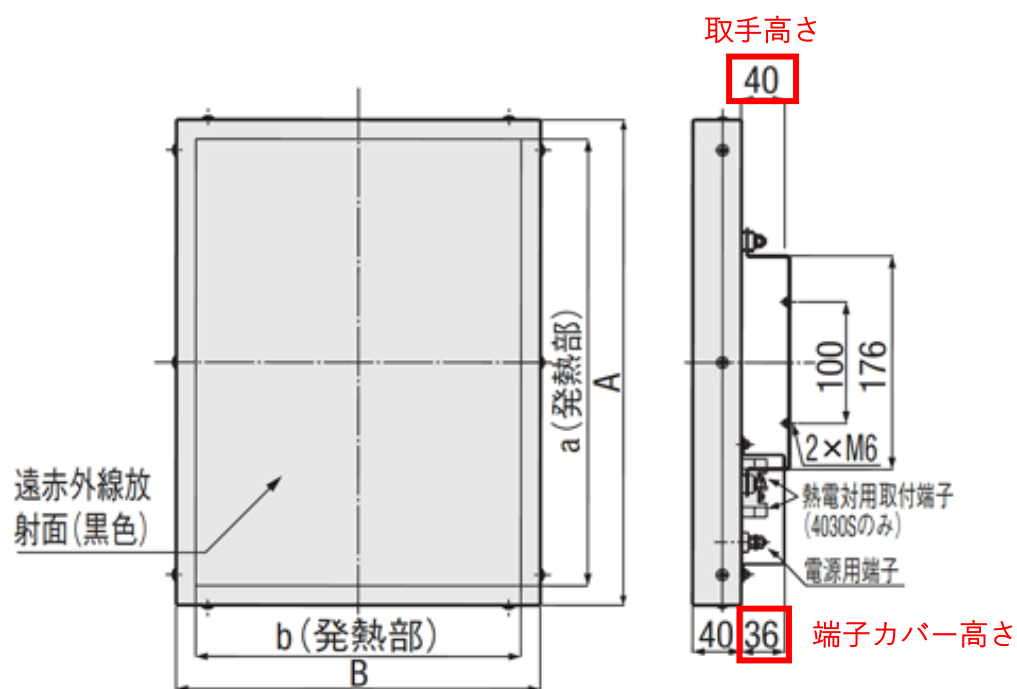
図 1 : 外形図 修正前
