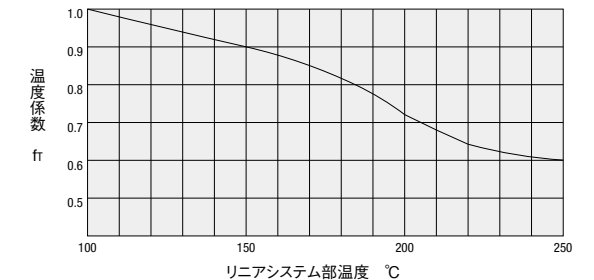
図-2. 温度係数
