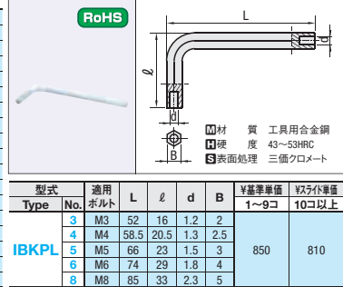
専用レンチ
