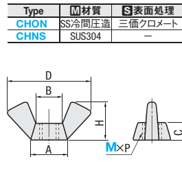
蝶ナット
