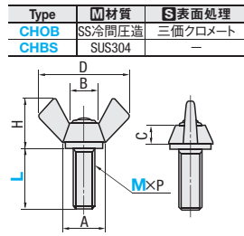
蝶ボルト
