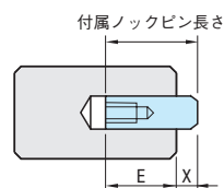
■サポートピラーノック穴付ー セット例
