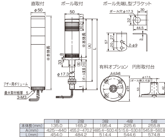
MST-LE-02*** (Φ50)
