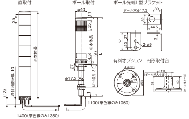
MST-LCE-02A*** (Φ40)
