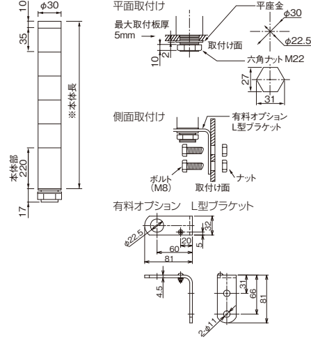
MST-MP-02 (Φ30)
