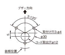
MST-LCE-02A*** (Φ40)
