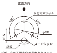
MST-LE-02*** (Φ50)
