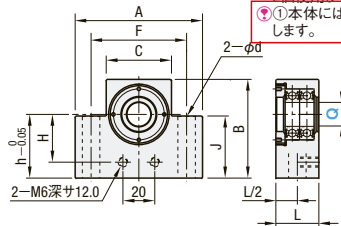
■コンパクトポジションインジケータ取付用セット品 MTWZ-CP 回転止め機能付
